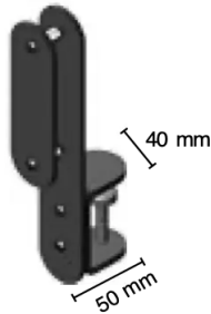
Tischklemme (einseitig) zur Befestigung der Trennwand an einem Arbeitstisch
