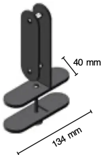
Tischklemme (zweiseitig) zur Befestigung der Trennwand zwischen zwei Arbeitstischen
